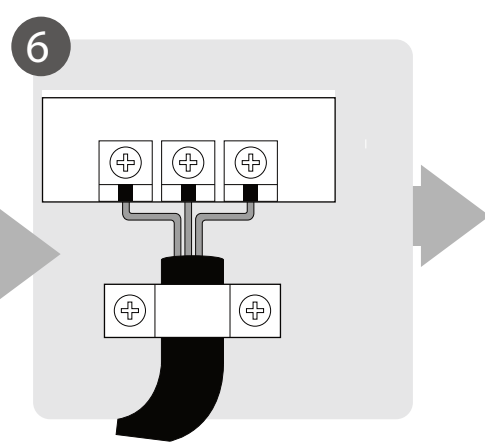
6 Conecte el cableado (no aplicable para algunas ubicaciones de Norte América)
