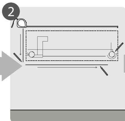
2 Determine la posición del agujero en la pared
